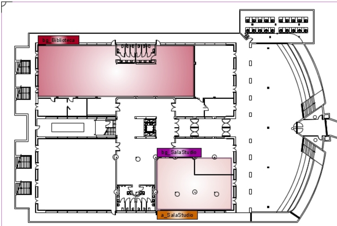
Piano Terra Biblioteca – Sala Studio
