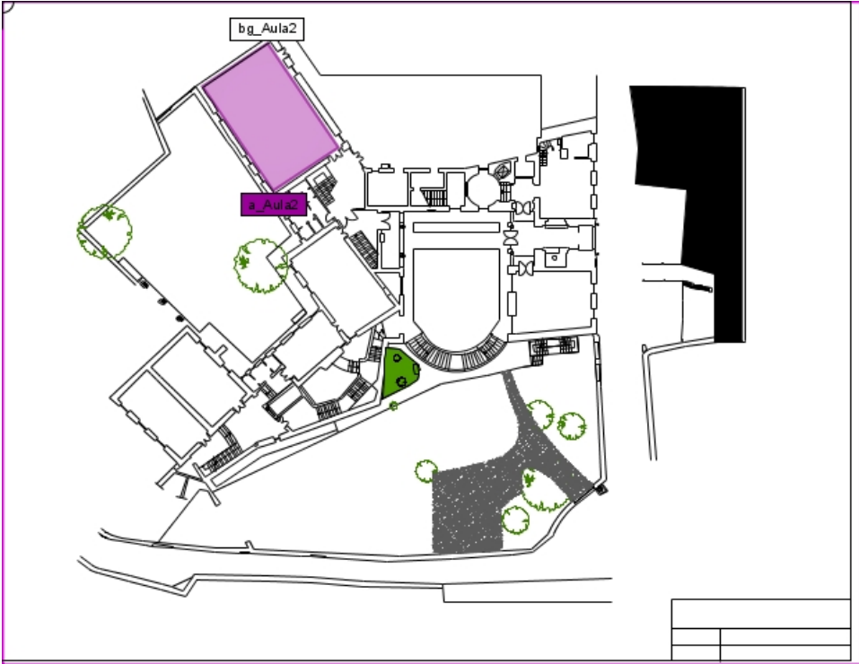
Piano Terra Aula 2
