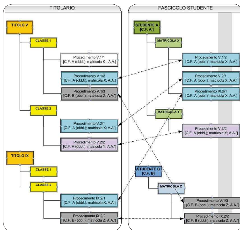
Lo schema logico del fascicolo elettronico dello studente UNINA
