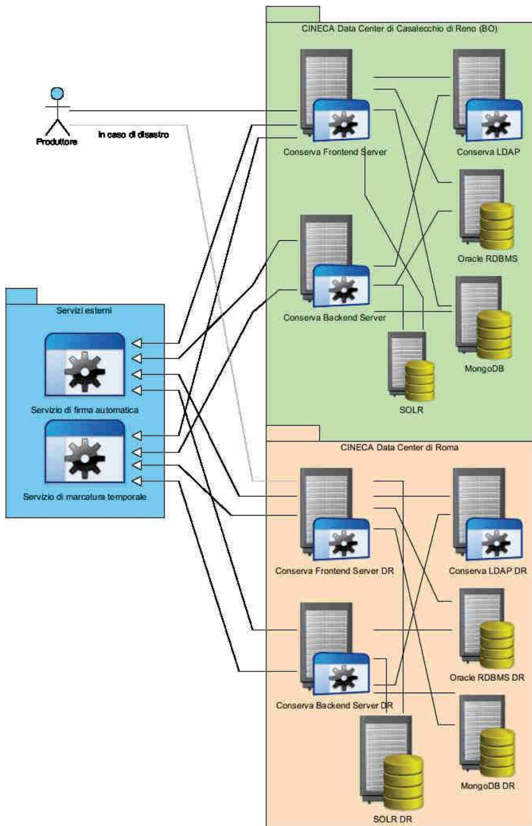
Figura 5 - Distribuzione topologica delle componenti fisiche di Conserve
