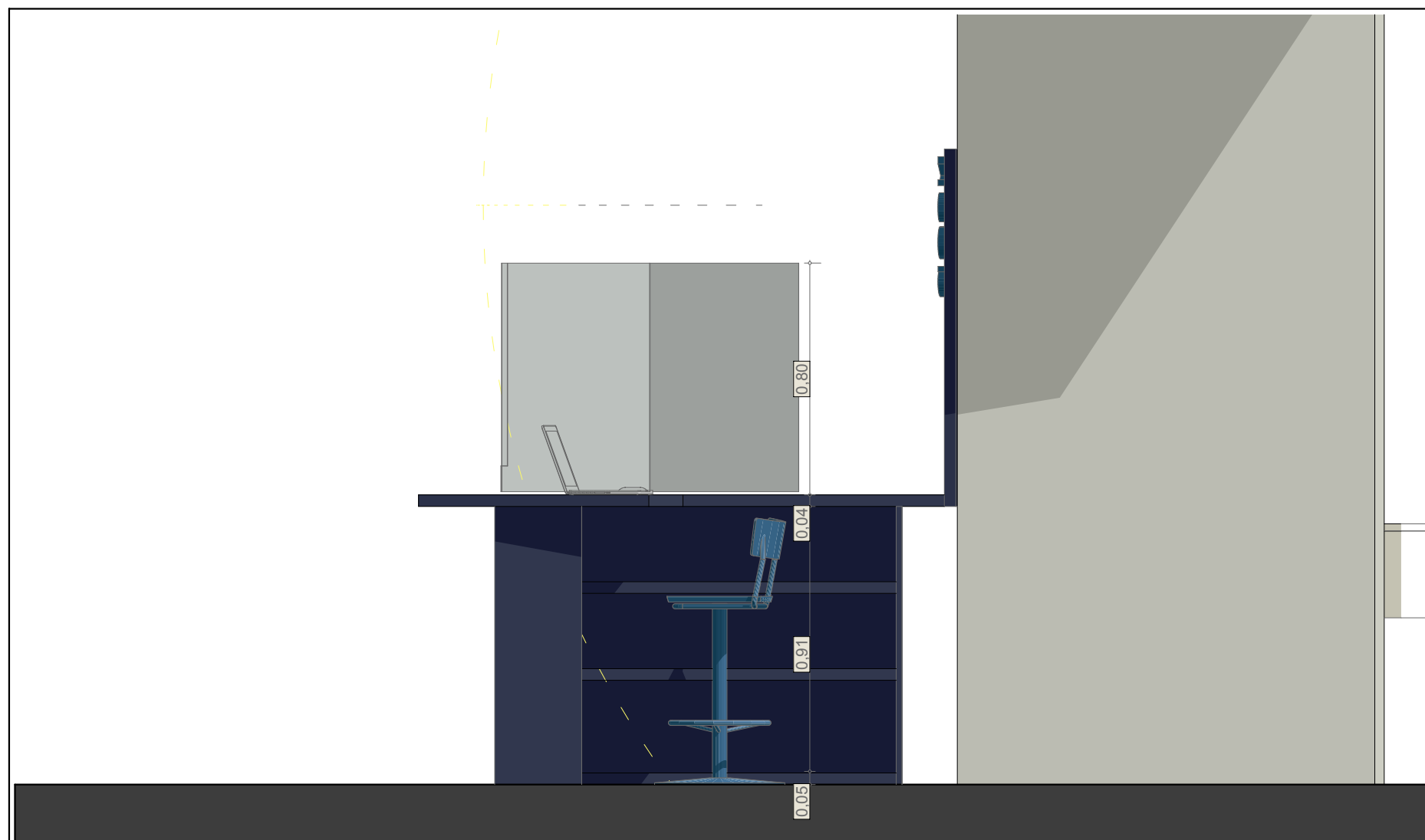
16 | SEZIONE 02 (8) (1:20)
